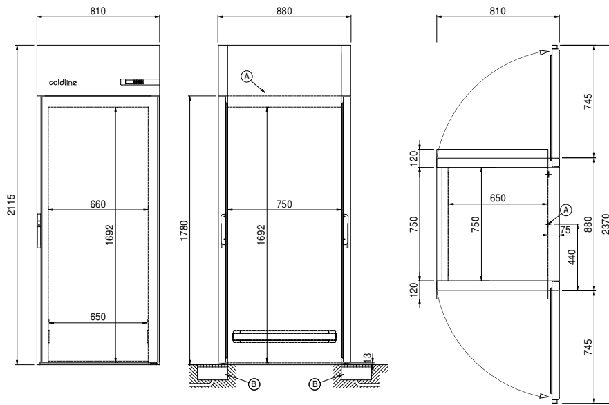
A: Sortie cable d'alimentation B: Condensation de vidange
